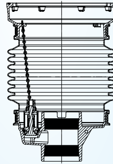
5 Gallon Fill or Vapor Spill Bucket
