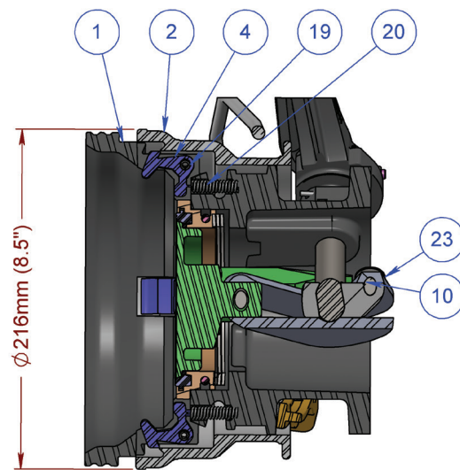
Seccion B-B
